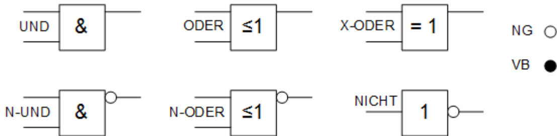
Abbildung 1: Logik-Symbole
