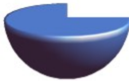
Abbildung 19: Halbkugel mit einem Endwinkel von 270°
